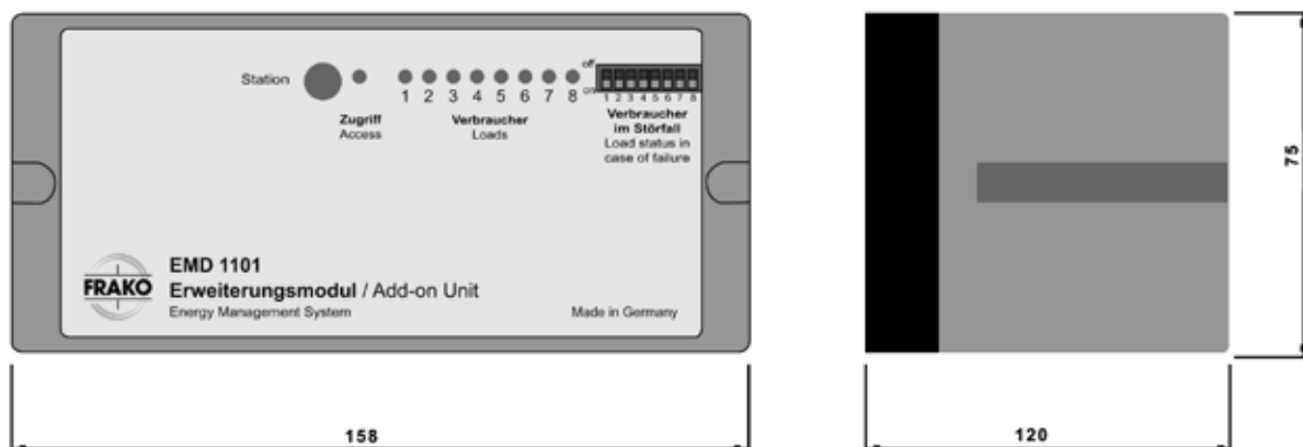
Maßbild EMD 1101
