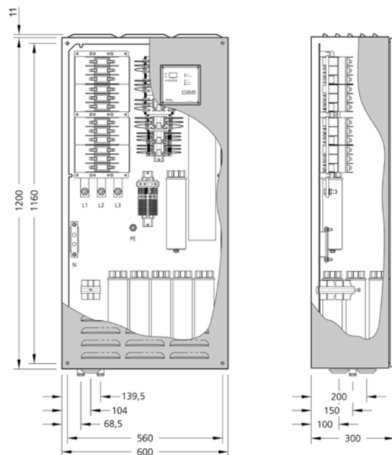
Maßbild LSK-3 (112,5 bis 200 kvar)
